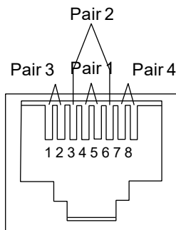
T568A
