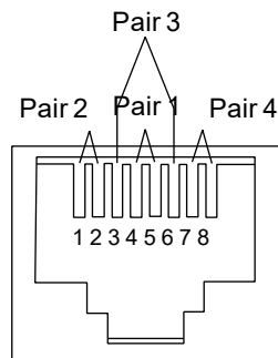
T568B
